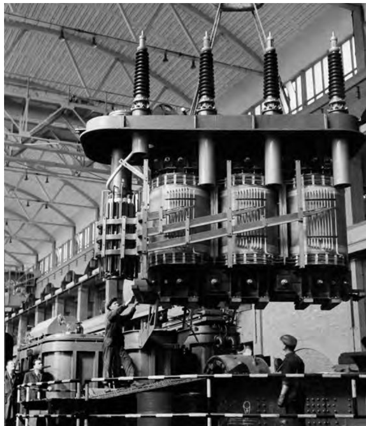
Detalj iz proizvodnje transformatora u tvornici Rade Končar, presnimka fotografije, Zagreb, 1954. / Muzej grada Zagreba
