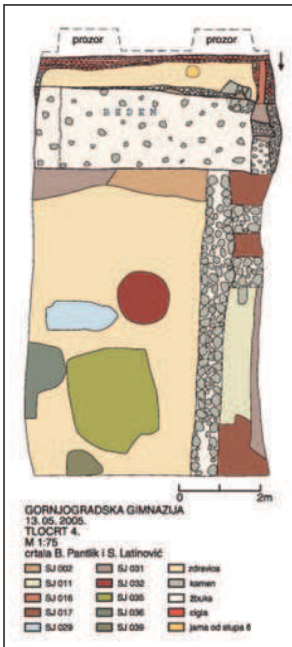
Gornjogradska gimnazija, kompozitni tlocrt (izradila: B. Pantlik, S. Latinović)
